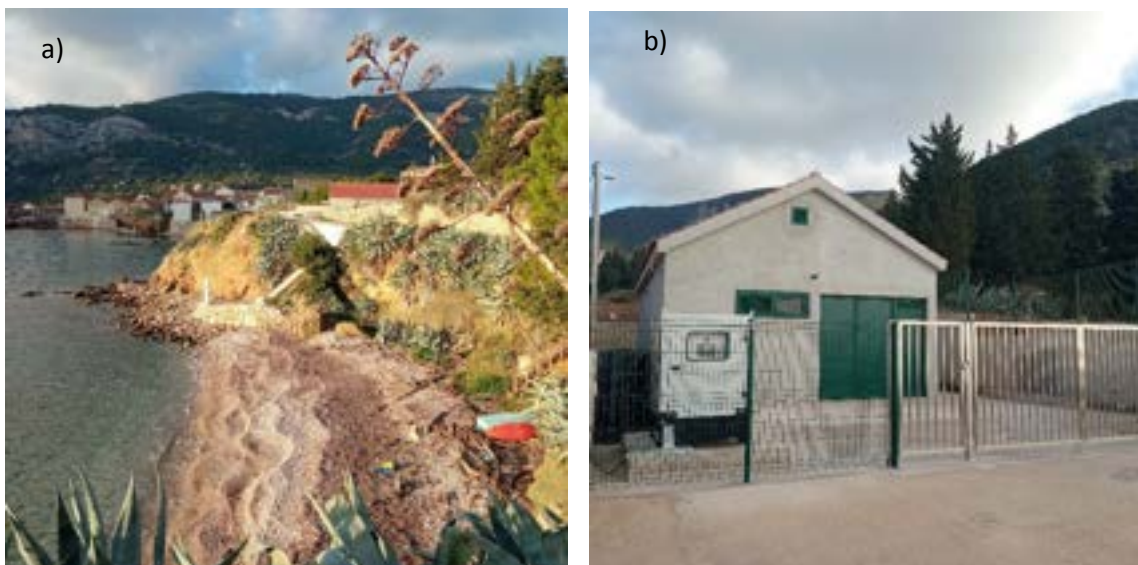
Slika 8. Radovi na izgradnji kanalizacijske infrastrukture, stanje 20.12.2022.: a) plaža za pse, b) objekt sustava za pročišćavanje otpadnih voda.
