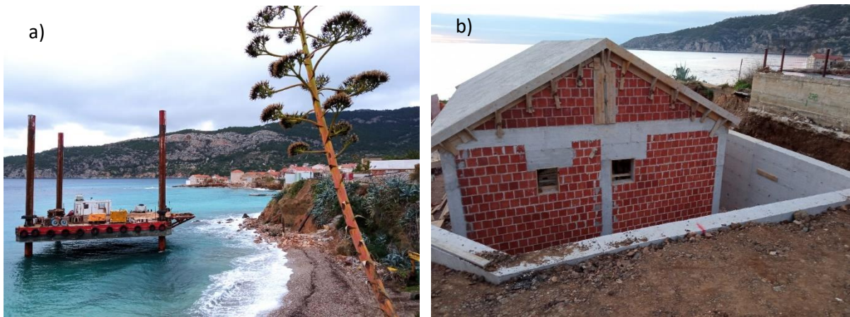
Slika 8. Radovi na izgradnji kanalizacijske infrastrukture, stanje 04.12.2021.: a) polaganje podmorskog ispusta, b) objekt sustava za pročišćavanje otpadnih voda.
